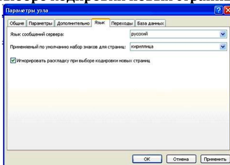
Рис.5. Настройка кодировки языка сайта в окне Параметры узла .
